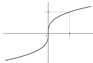
OBRÁZEK 3. Graf funkce třetí odmocnina
