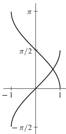
OBRÁZEK 9. Grafy funkcí arkussinus a arkuskosinus
