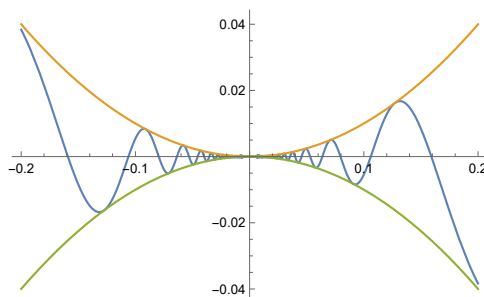
OBRÁZEK 13. Graf funkce z Příkladu 5.8.2
