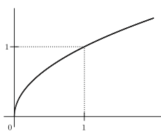
OBRÁZEK 2. Graf funkce druhá odmocnina
