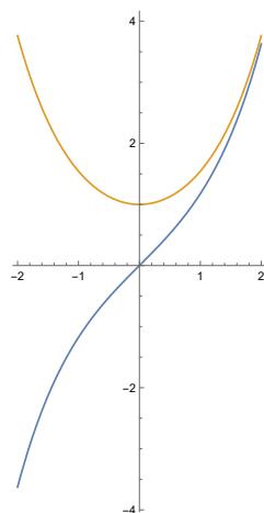
OBRÁZEK 14. Graf hyperbolického sinu a cosinu
