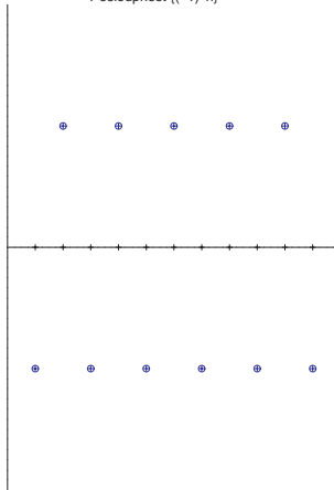
Posloupnost \{(-1)^n\}
