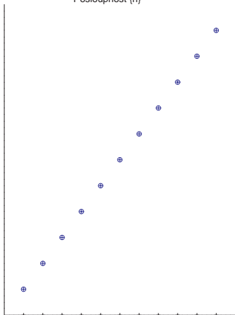
Posloupnost \{n\}
