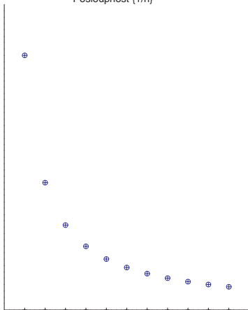
Posloupnost \{1/n\}
