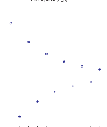
Posloupnost \{P_n\}
