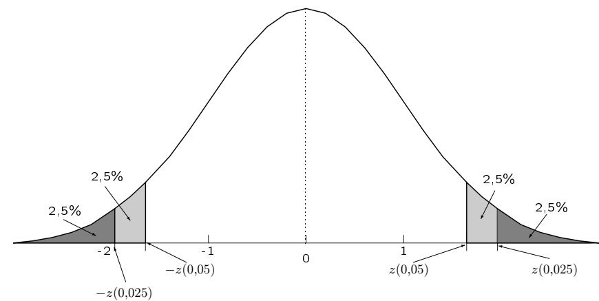
Hustota Z za platnosti H_0
