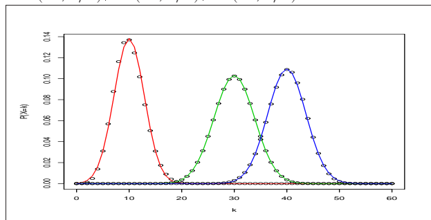
bi(60, 1/6), bi(60, 3/6), bi(60, 4/6)
